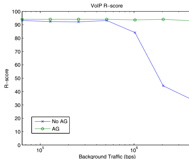
Fig. 8 VoIP R-score
